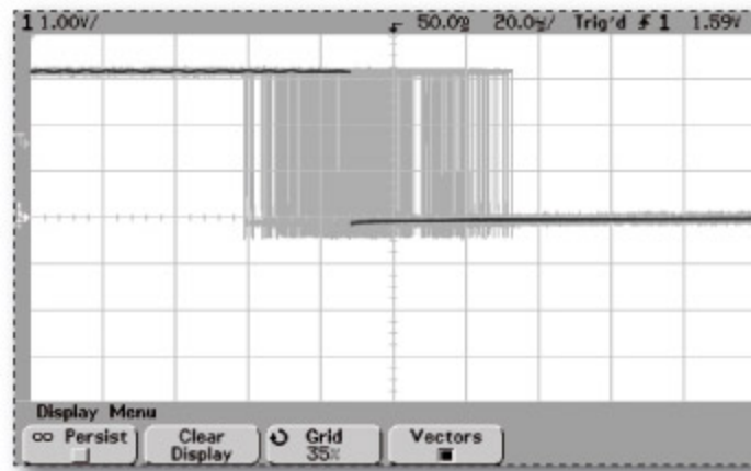
Fig. 9 : Exécution de xenomai_square en mode utilisateur
