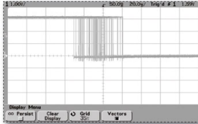
Fig. 10 : Exécution de xenomai_square_module en mode noyau
