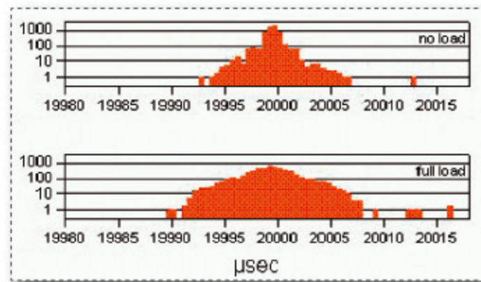
Fig. 3 : Représentation sur un système temps réel
