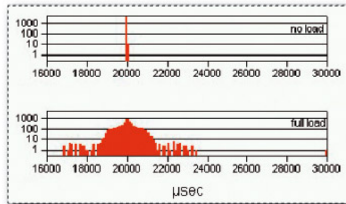
Fig. 2 : Représentation sur un système classique
